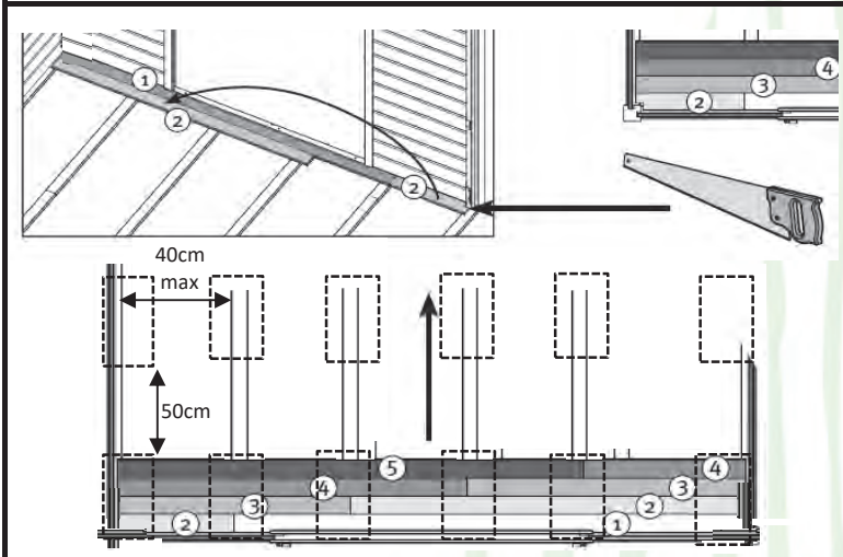
UŁOŻENIE BLOCZKÓW BETONOWYCH POD KONSTRUKCJĄ PODŁOGI/DOMKU
